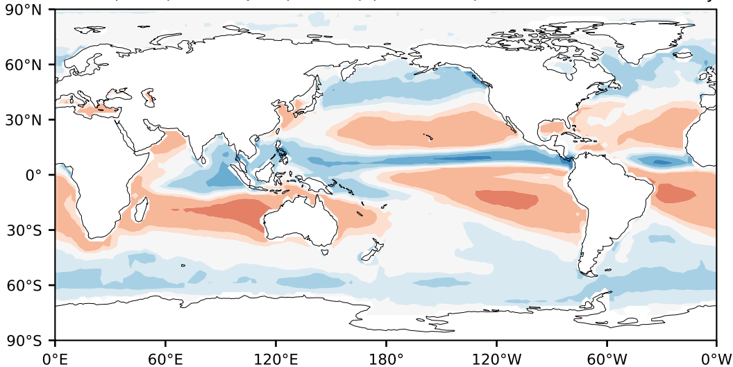
PRECT(GPCP) minus QFLX(OAFLux) (1979-2013)
